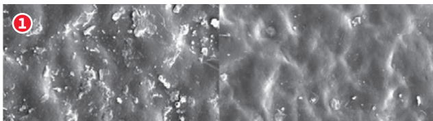
1 Kunststoffoberfläche: Vor der Reinigung / Nach der Reinigung Plastic Surface: Before Cleaning / After Cleaning 200:1
