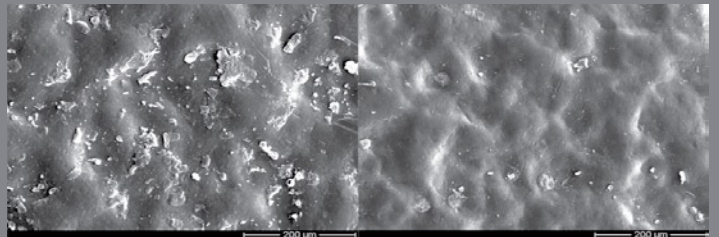
Kunststoffoberfläche: Vor der Reinigung / Nach der Reinigung Plastic Surface: Before Cleaning / After Cleaning 200:1
